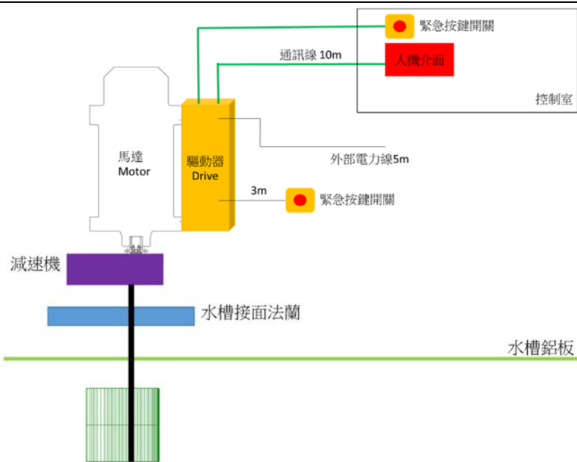
圖 2. 擺動翼水槽安裝與相關機電示意圖
